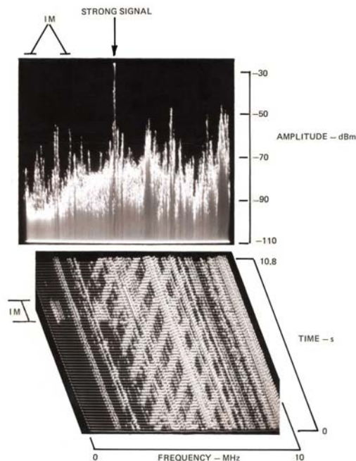
Figure 7 In-Band IM Noise
